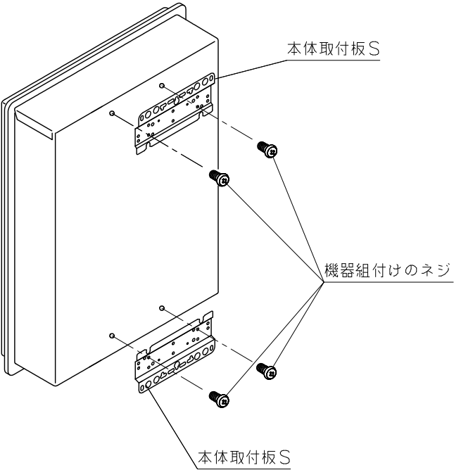
■ 取付参考図
