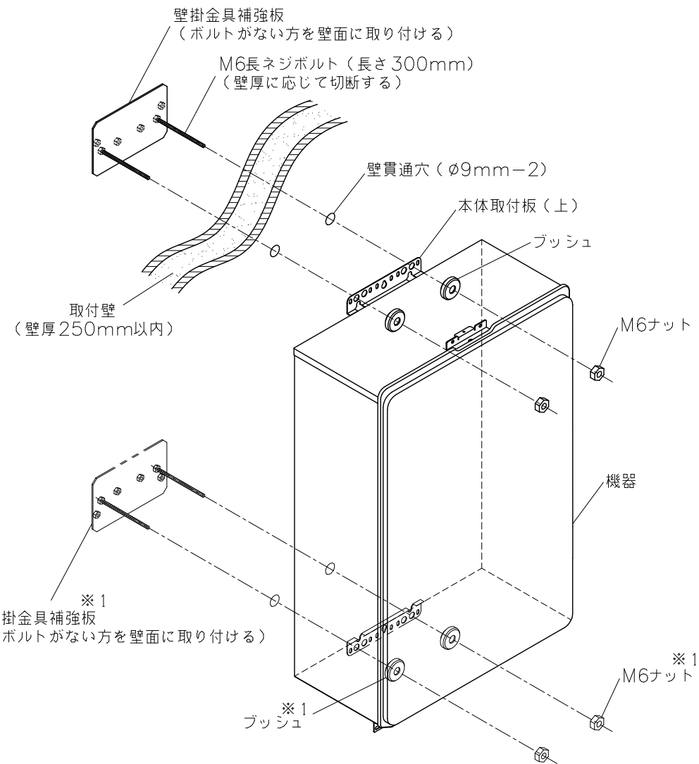
■ 取付要領図
