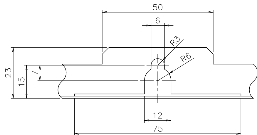
■A部詳細 (尺度 1/1)
