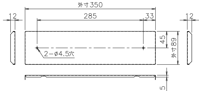
■ PS化粧板
