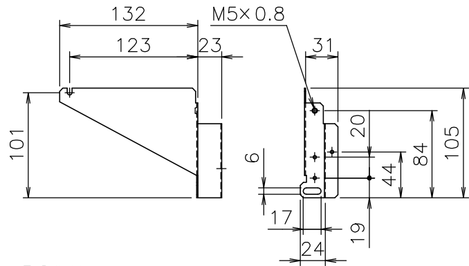
■ PS化粧板
