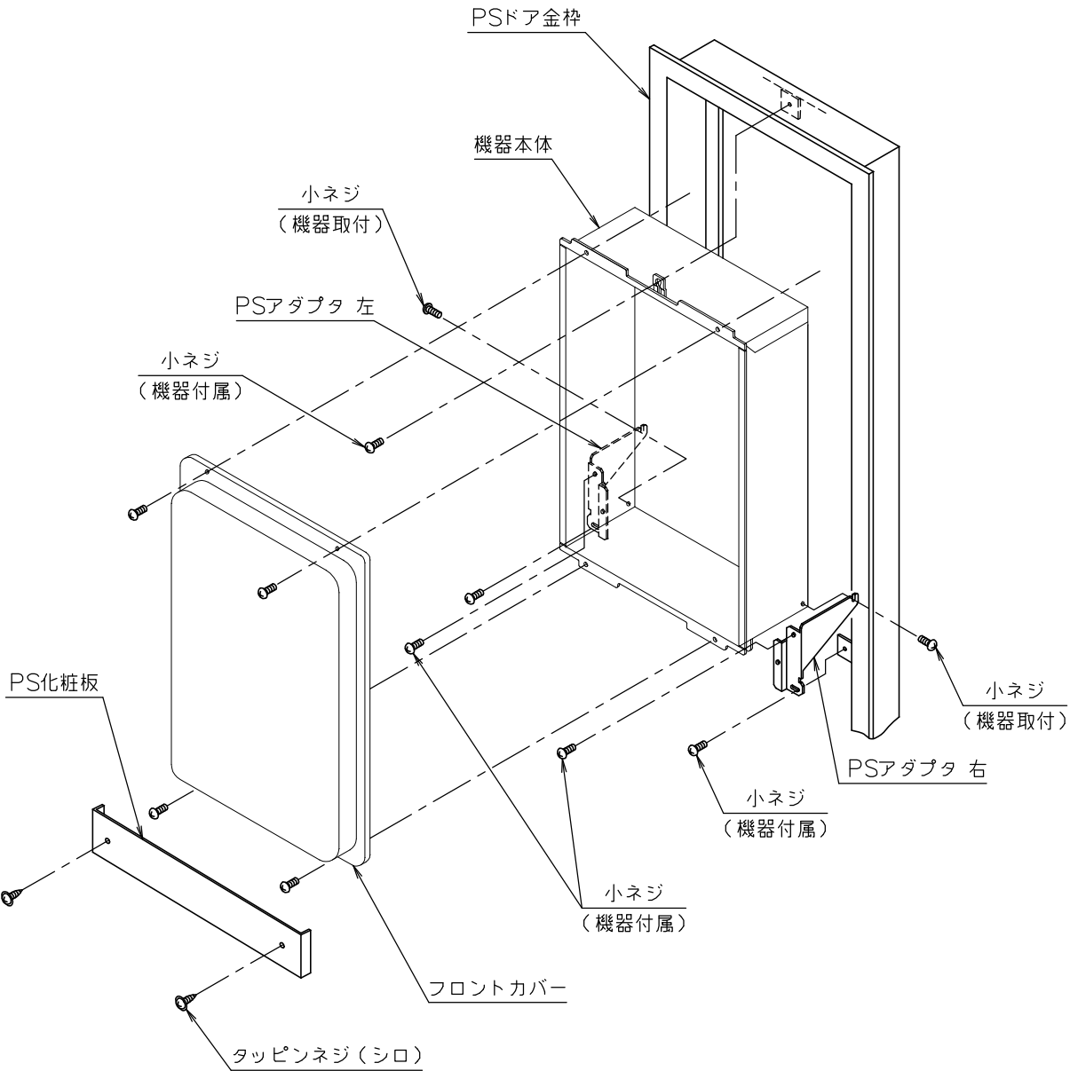
■ 取付参考図
