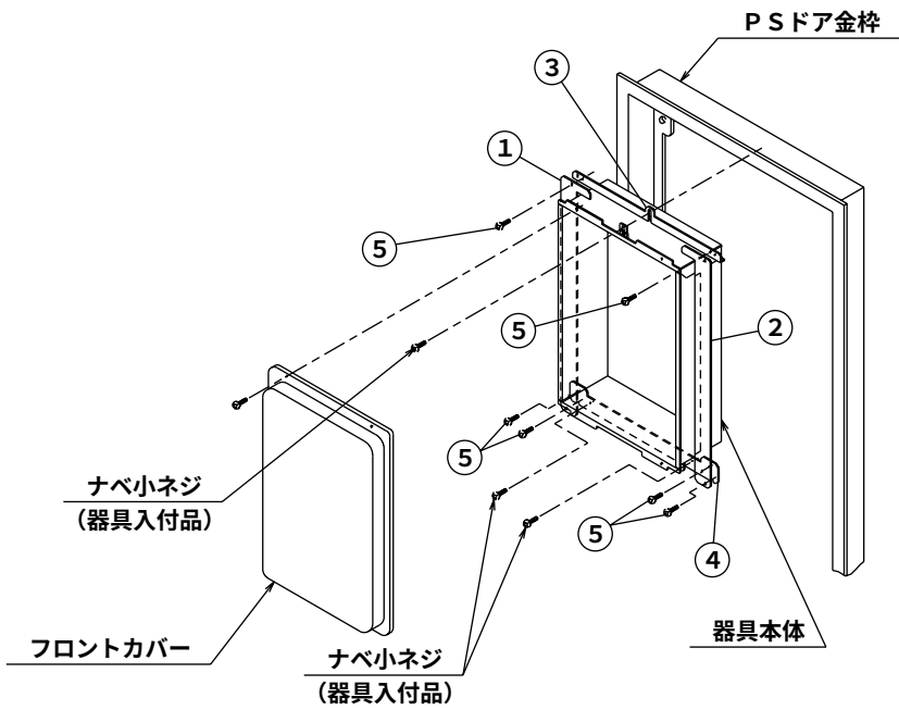
取付完成図（概略）
