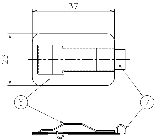
A部（⑥,⑦の外形視）詳細（尺度1/1）
