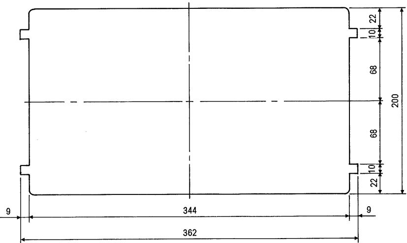
⑥ BUAユニットバス用しゃ熱板A
