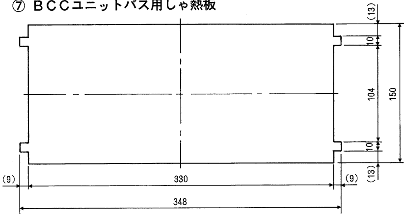
⑦ BCCユニットバス用しゃ熱板
