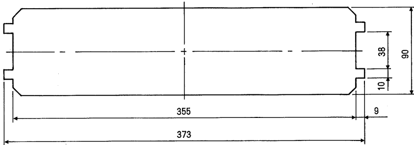
⑥ BUAユニットバス用しゃ熱板A
