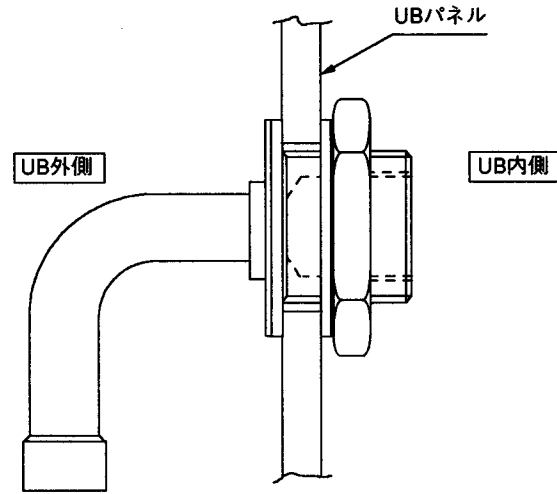
取付図
