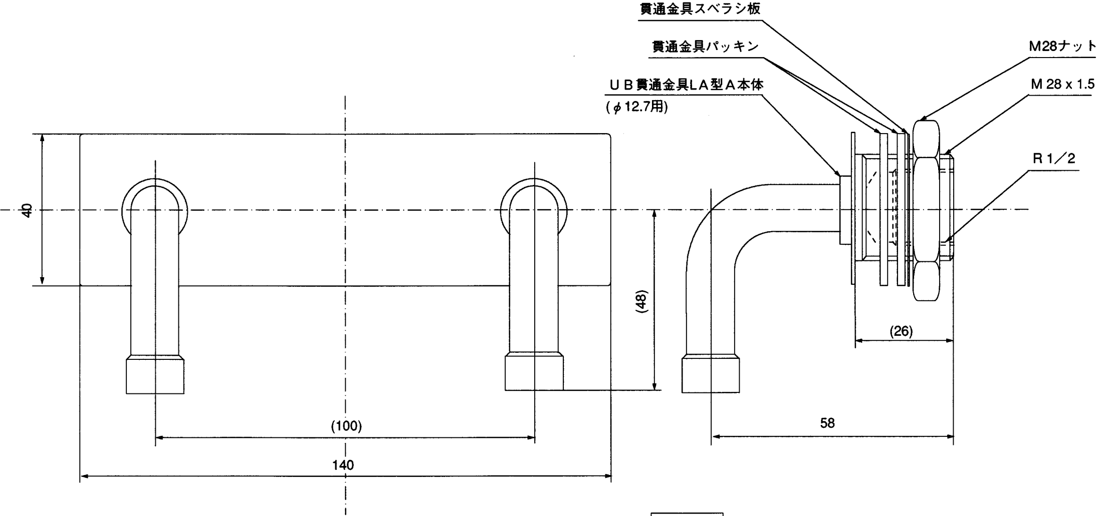
取付図
