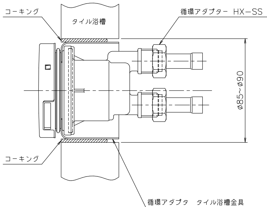
■取付図（循環アダプター HX-SSを取付けた一例です）
