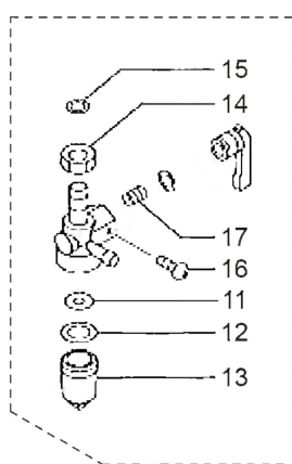
10 フューエルストレーナ詳細
