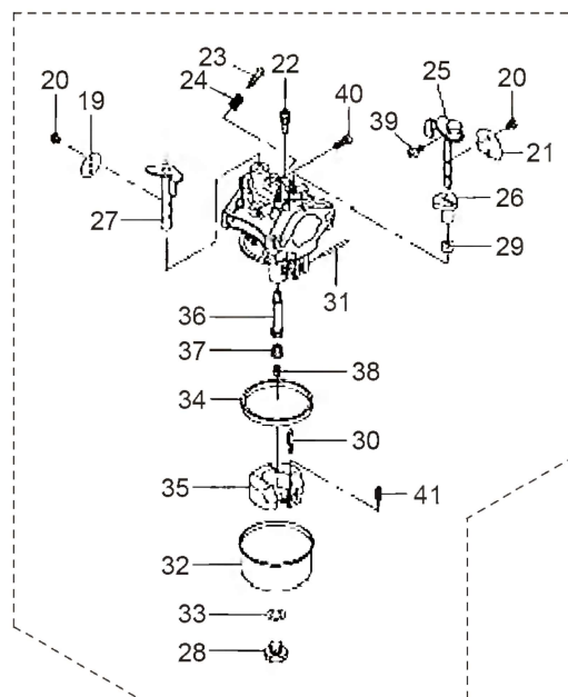
18 キャブレタ詳細
