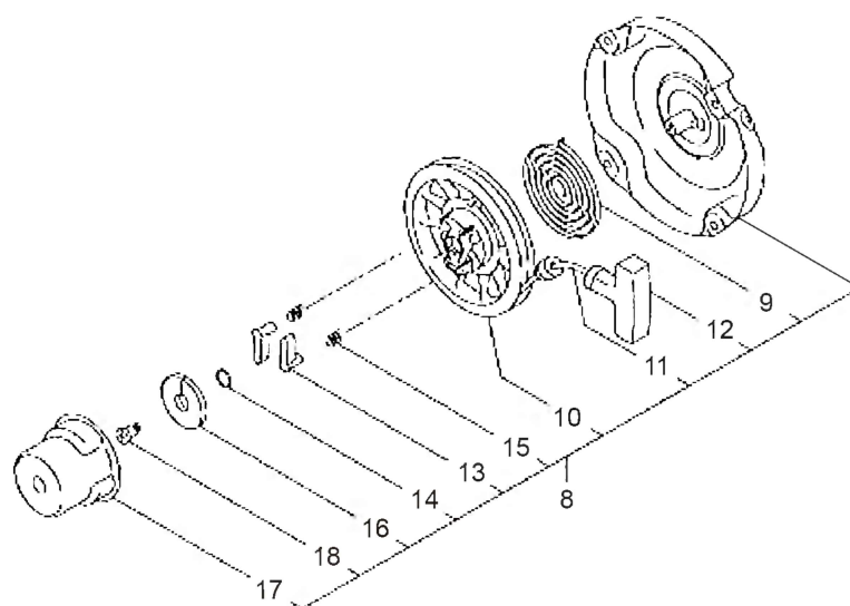
リコイルスターター詳細
