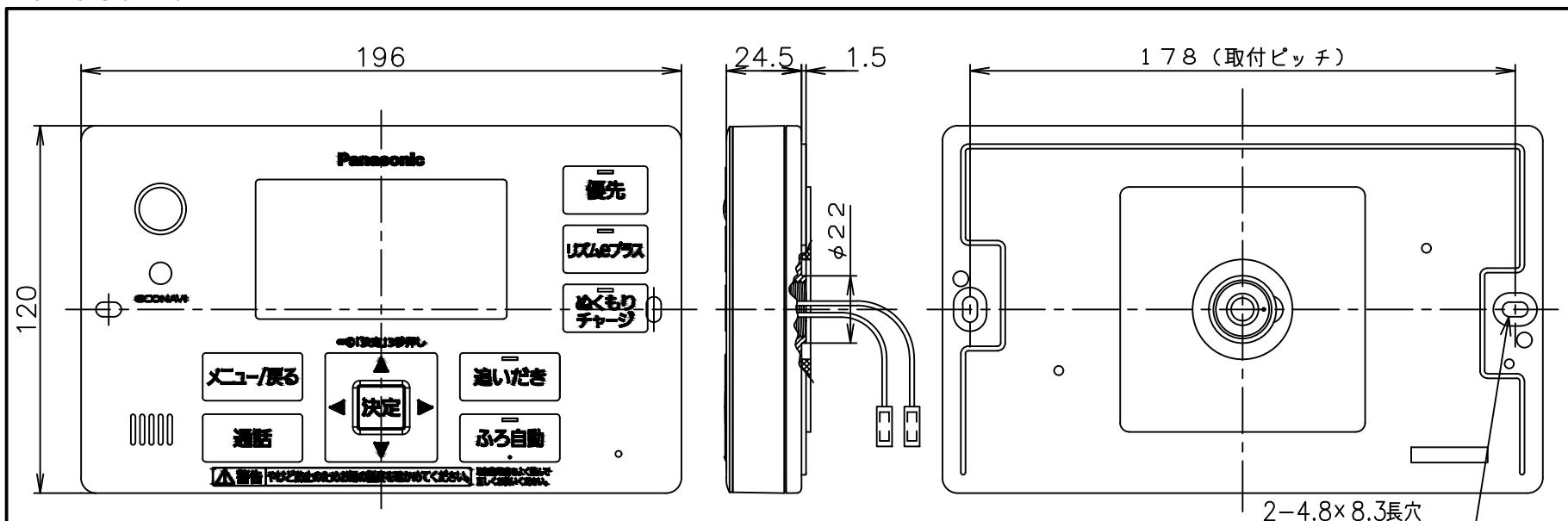
裏面図
