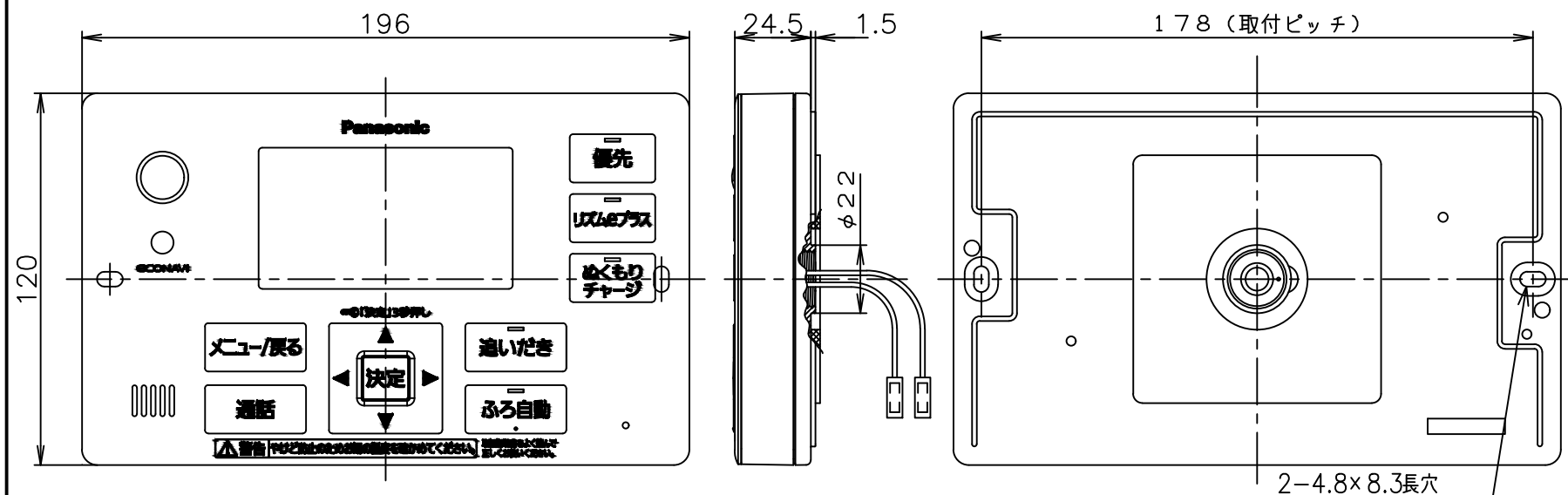
裏面図
