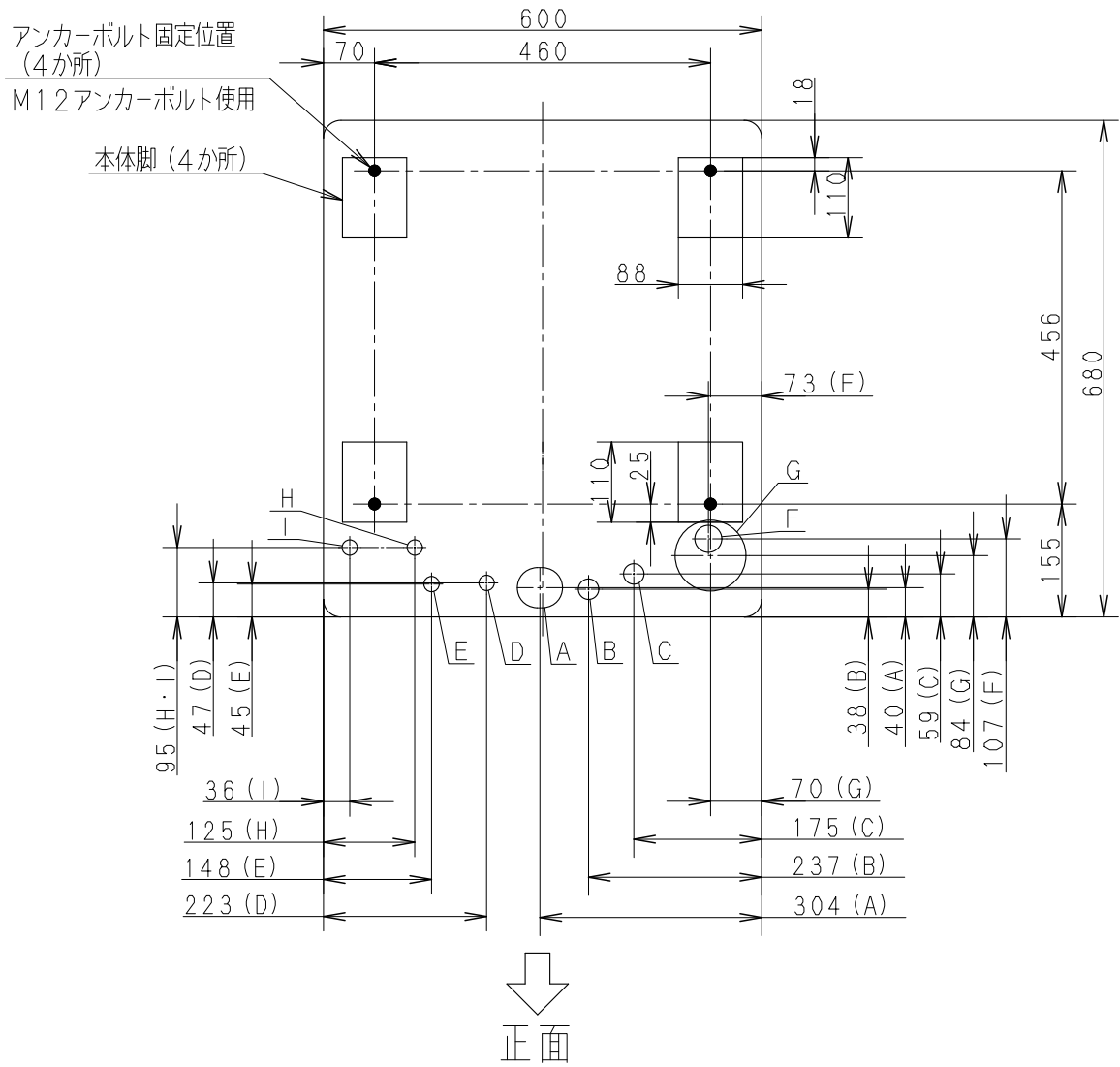
配管位置（底板上上面図）
