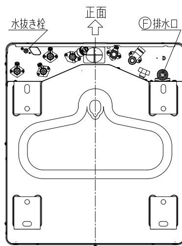
本体下から見た図
