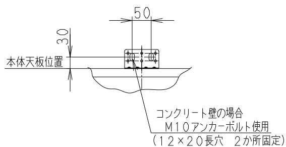
上部固定金具使用時固定詳細図
