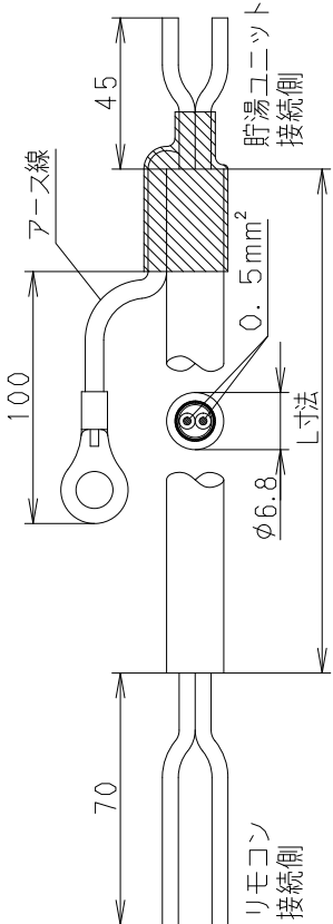
リモコンコード (別販品)
