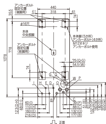
配管位置／アンカーボルト位置
