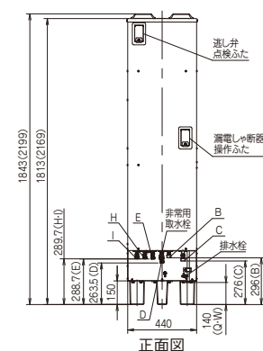
正面図
