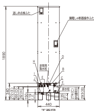
正面図
