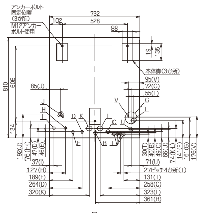
配管位置／アンカーボルト位置
