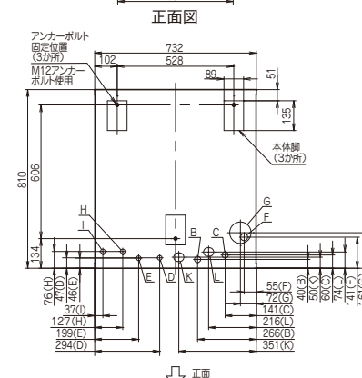
配管位置／アンカーボルト位置
