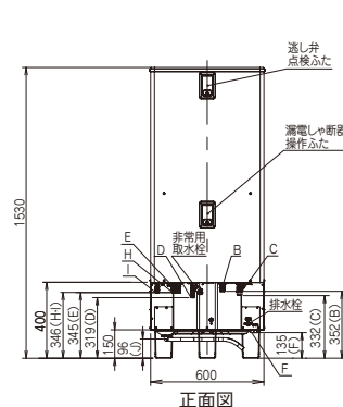
正面図
