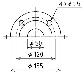
FLANGE SIZE フランジ寸法
