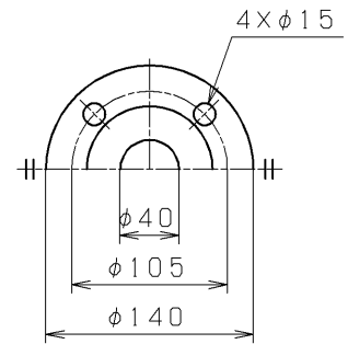
FLANGE SIZE フランジ寸法
