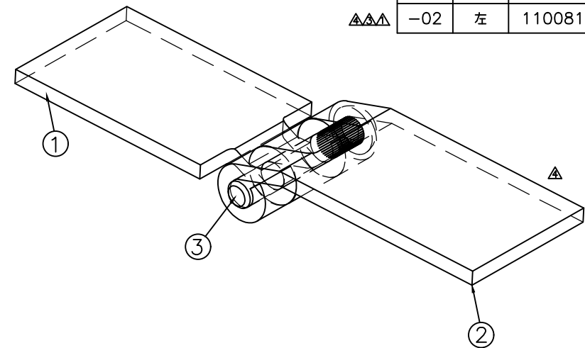
③ ローレットピン
