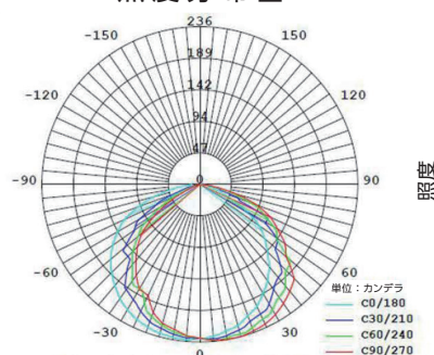
照度分布図
