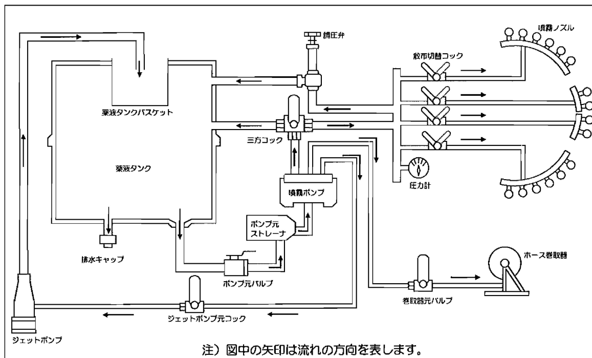
●配管系統図
