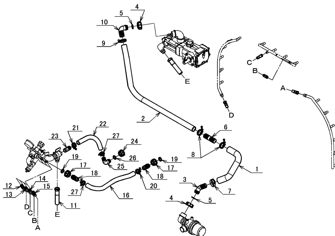
●配管系統図
