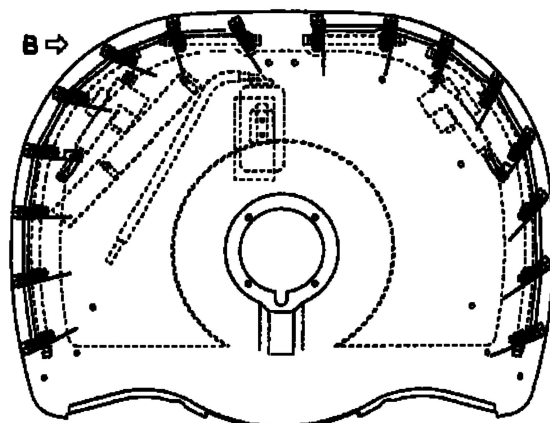
噴頭 後方より見る
