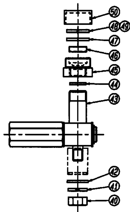
ノズル部詳細図
