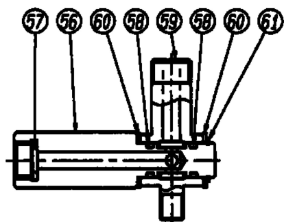
より戻し組立詳細図
