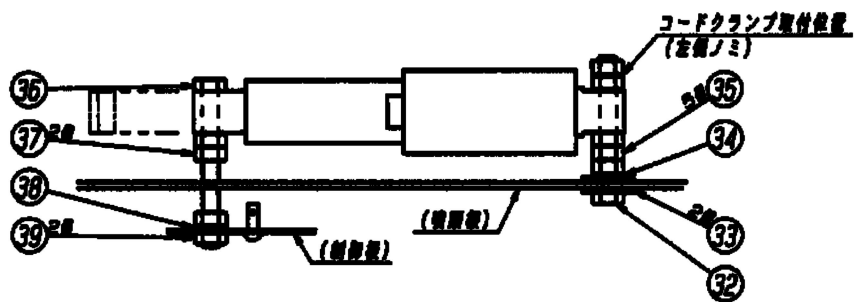
シリンダー取付部詳細図 (上より見る) (左右対称)
