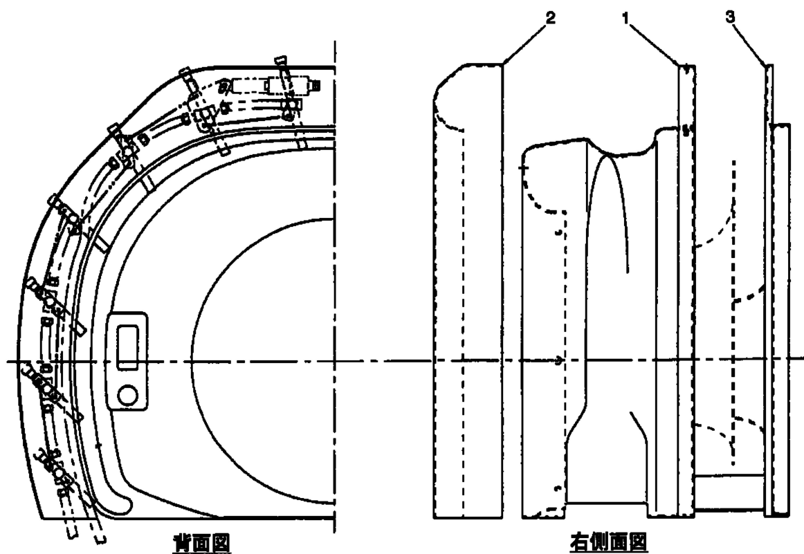
噴頭部概略図
