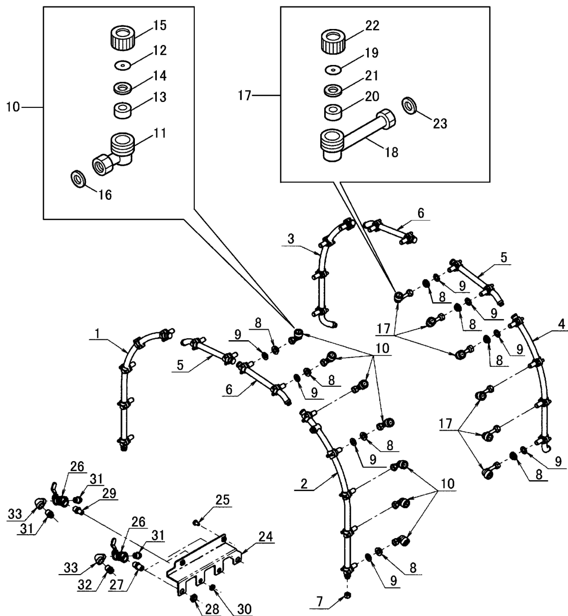
ノズル配列図
