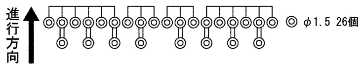
ノズル配列図
