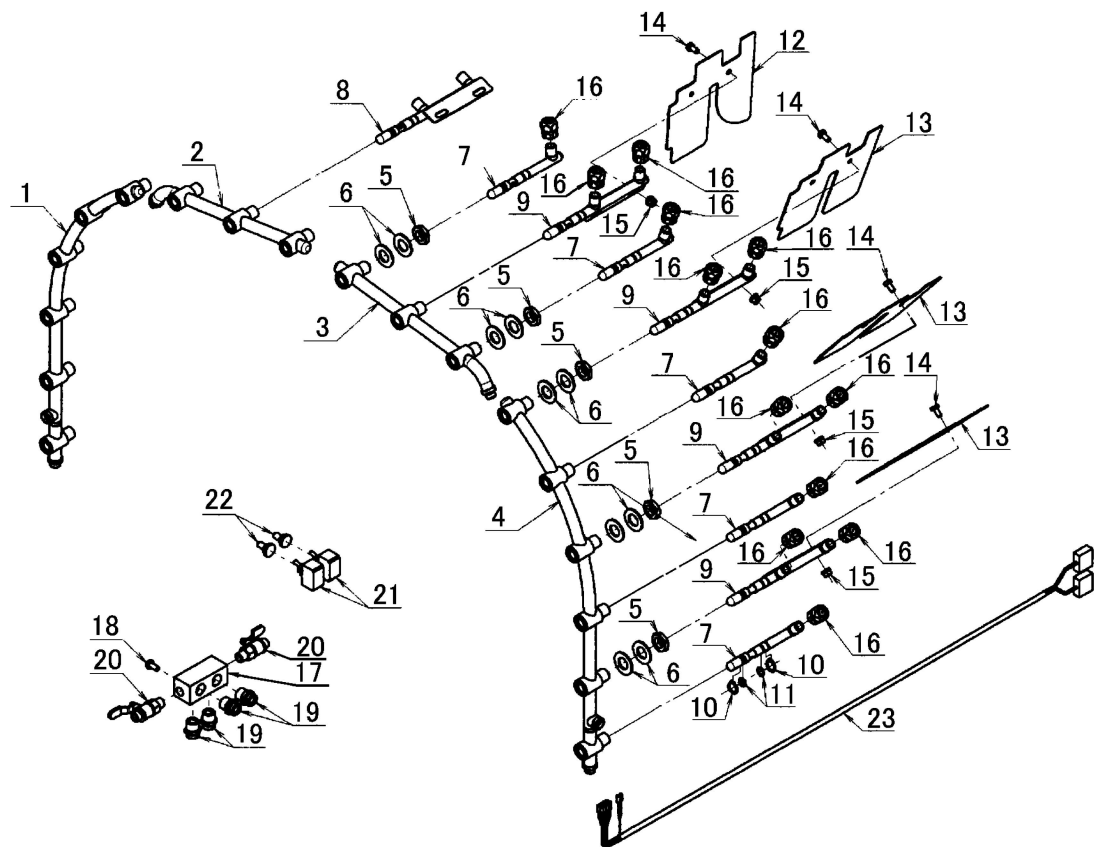
ノズル配列図
