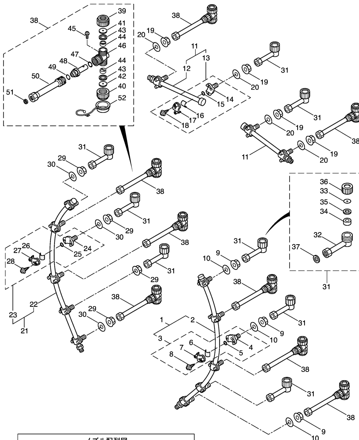
ノズル配列図
