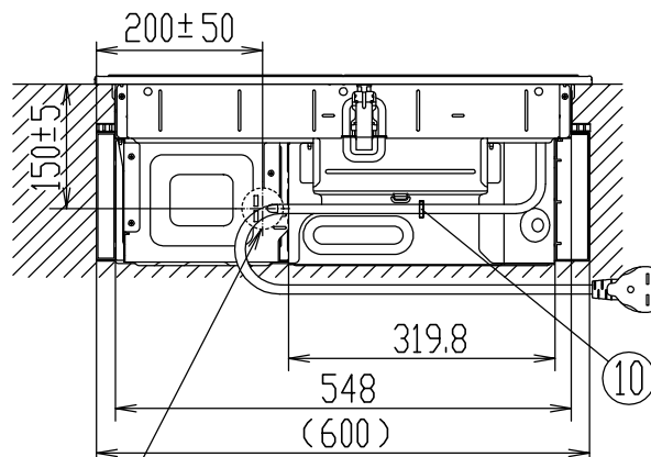
背面図
