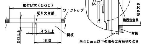
〈正面（断面）図〉
