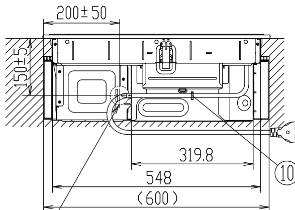
背面図
