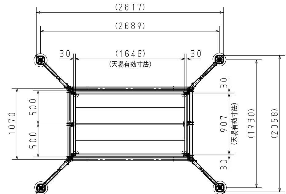
作業床
