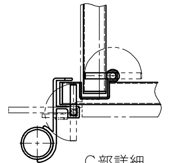
C部詳細 (S = 1 : 5)
