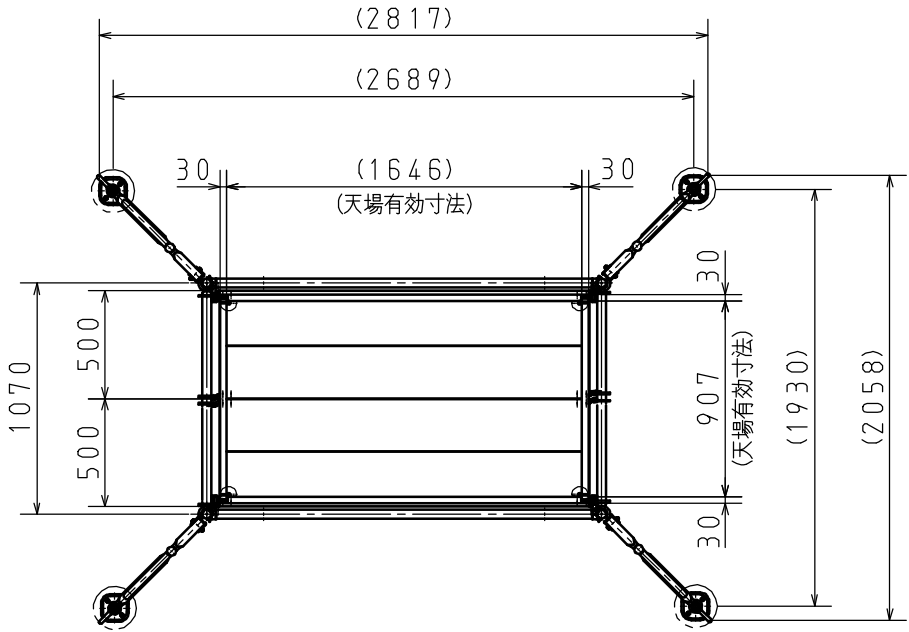
作業床
