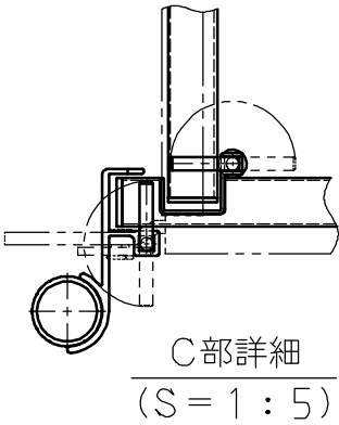
作業床
