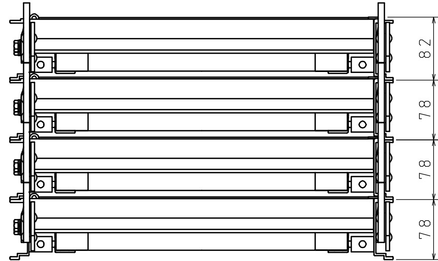
積み重ね状態 (S = 1 : 5)
