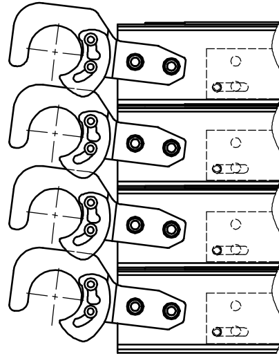
積み重ね状態 (側面) (S = 1 : 5)
