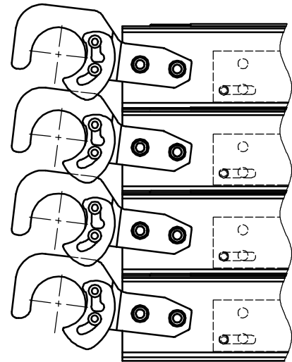
積み重ね状態 (側面) (S = 1 : 5)
