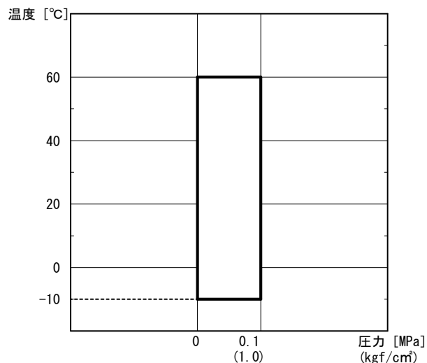
耐震ジョイントの使用範囲
