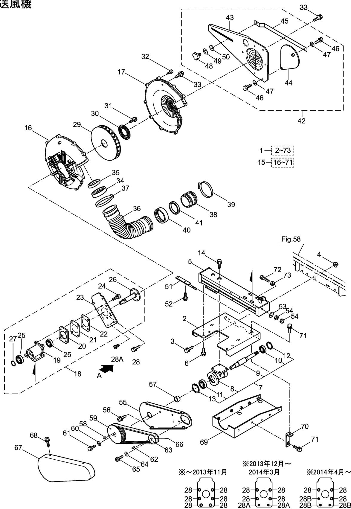
矢視A(取付ボルト詳細)
