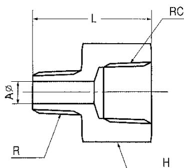
逆ブッシング R・Bu (REVERSE)
