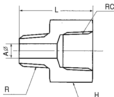
同径ブッシング E・D・Bu (EQUALISED DIAMETER)
