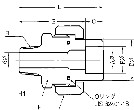
さし込み(内径)×ねじ込み(外径) UNION(b)
