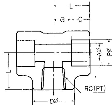
さし込み/ねじ込み SW×PT.TEE
