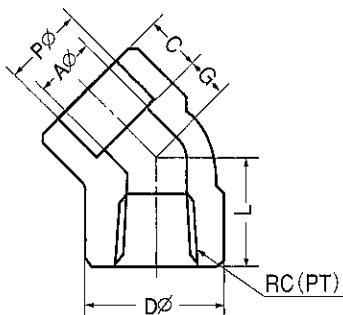
さし込み/ねじ込み SW×PT.45°E
