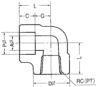
さし込み/ねじ込み SW×PT.90
