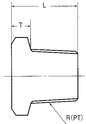
プラグ P
