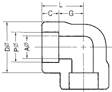
さし込み形 SWE
