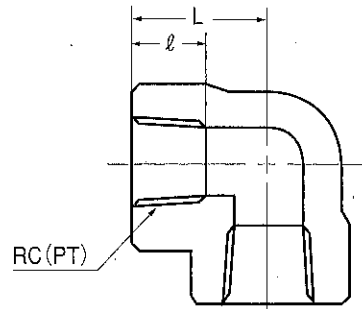
ねじ込み形 PTE
