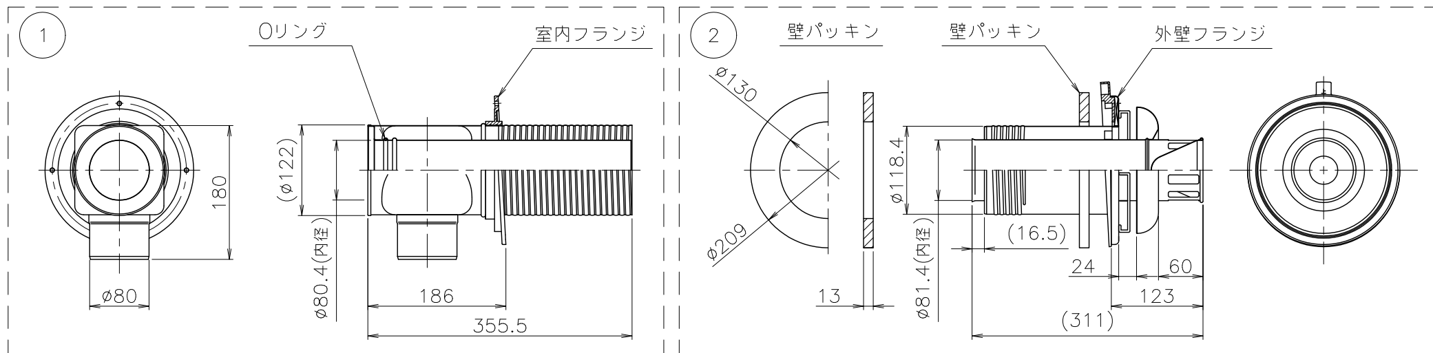
■側面図（組立）
