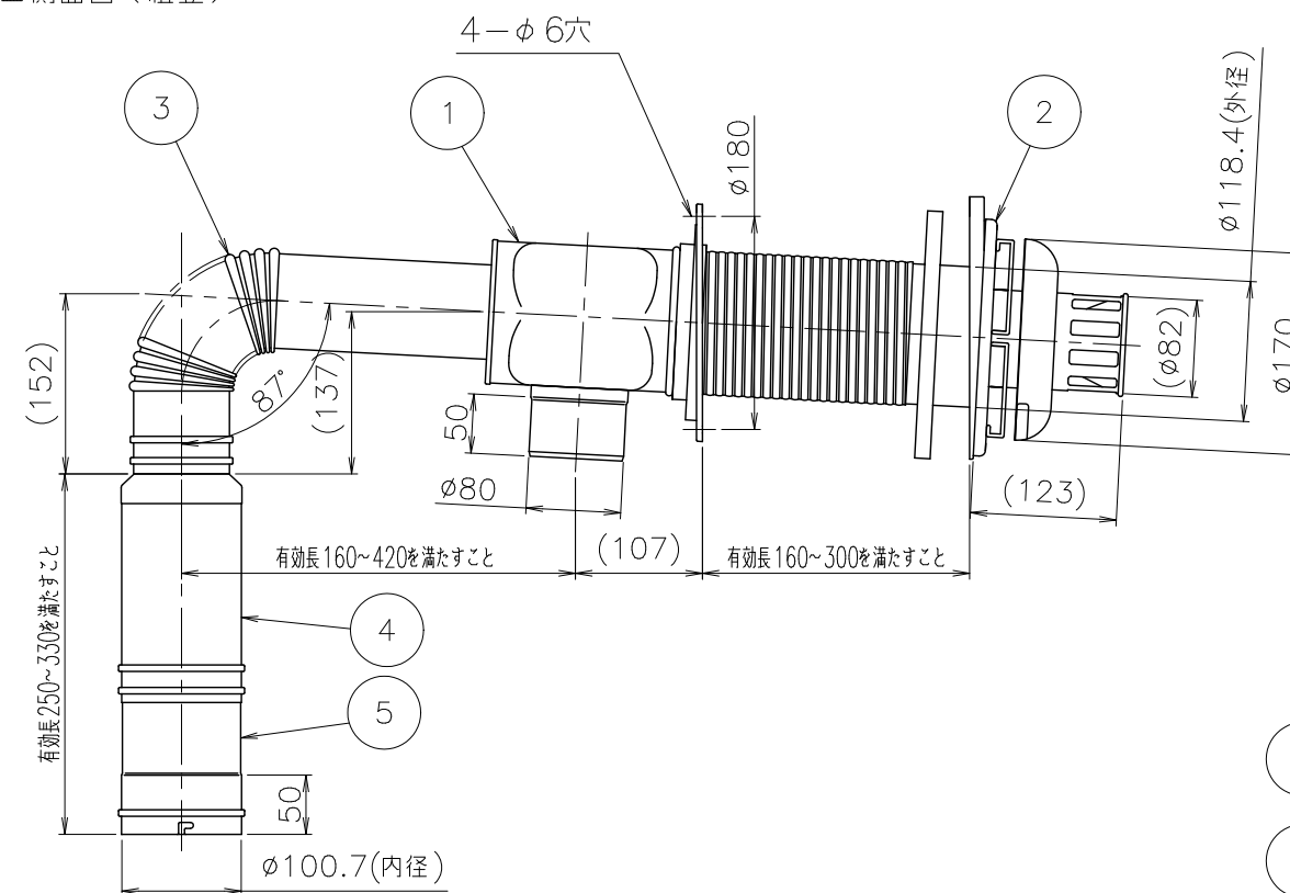
■側面図（組立）
