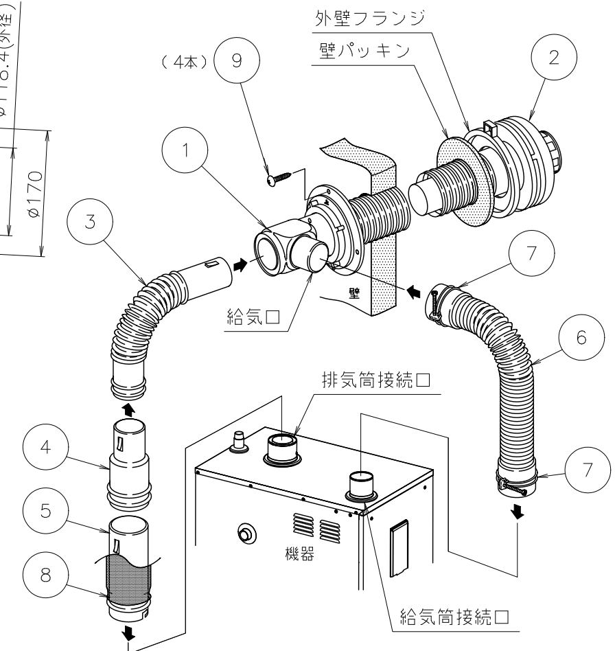
■ 取付要領図（概略）
