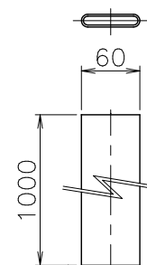
(8) 自然放置姿寸法
