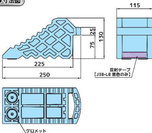
●寸法図
