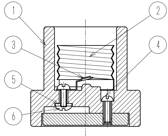
断面A-A
