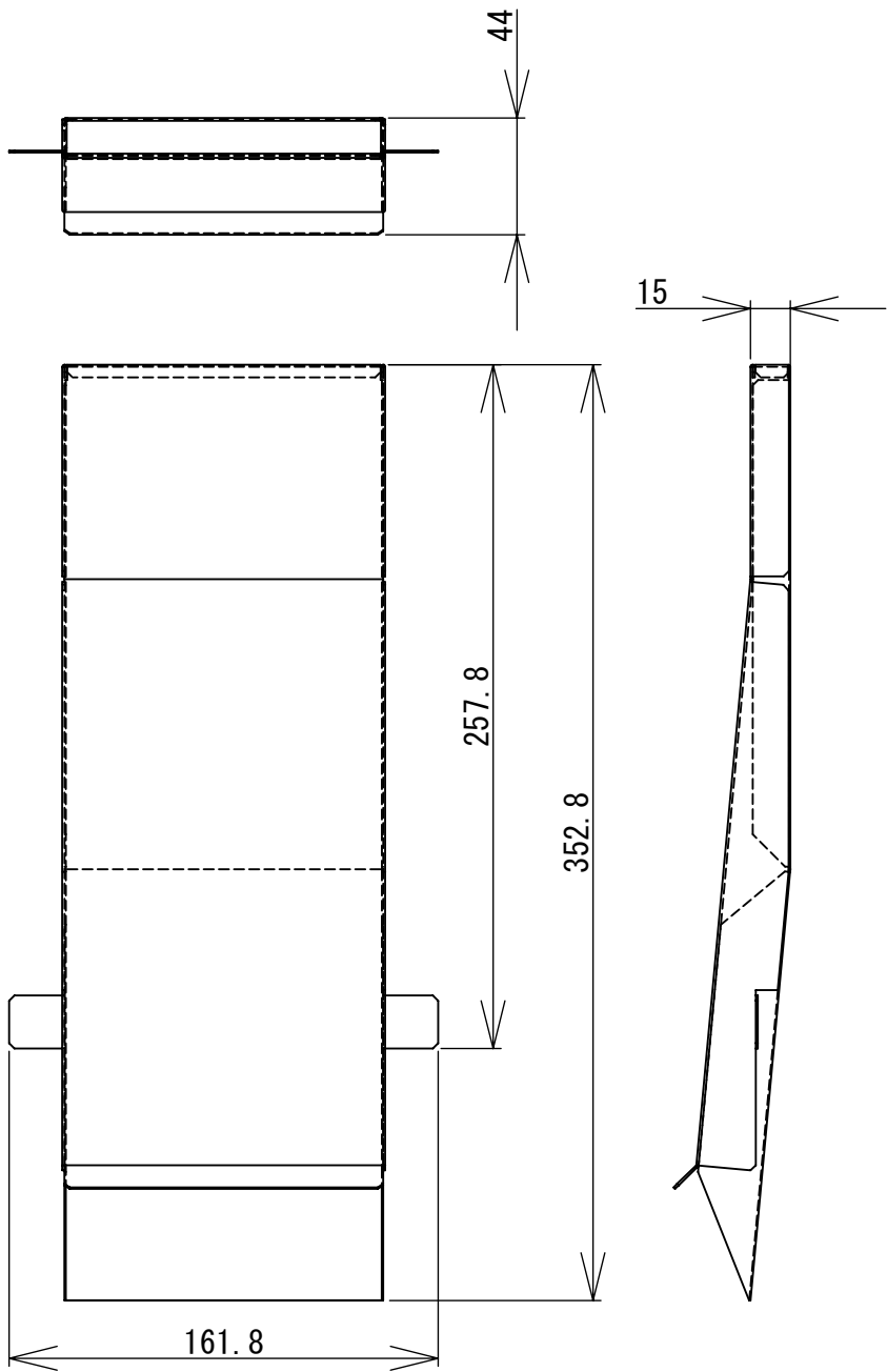
排気筒
