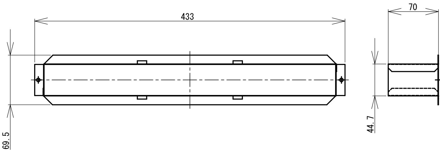
中間排気筒
