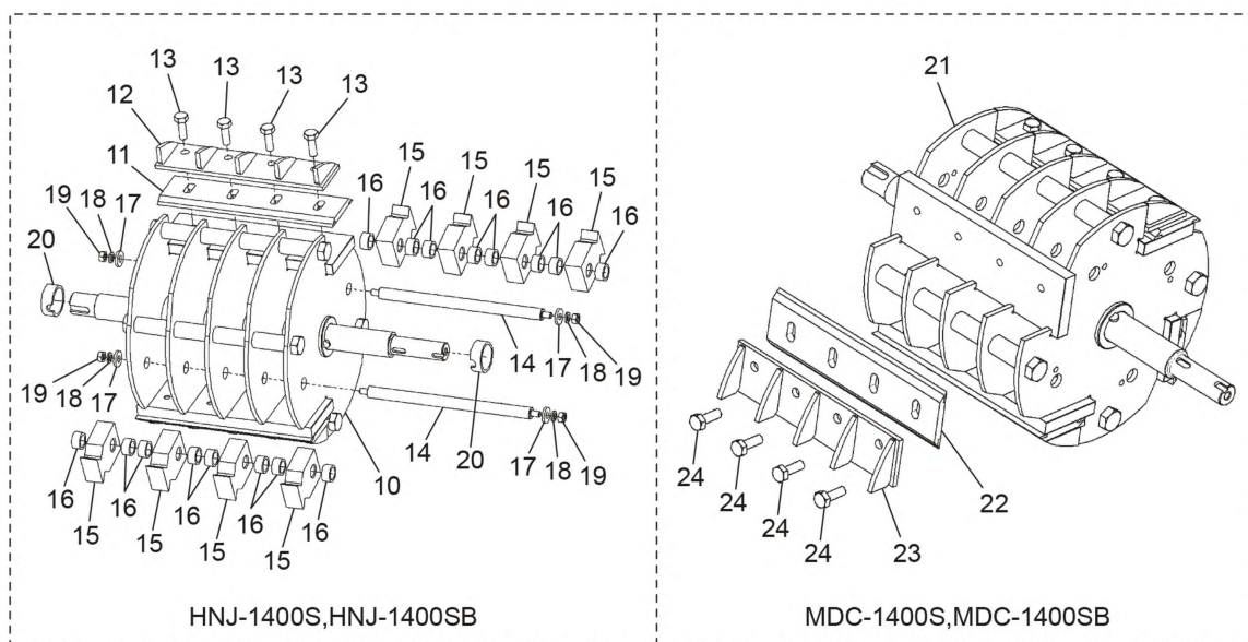
複合ロータ詳細
