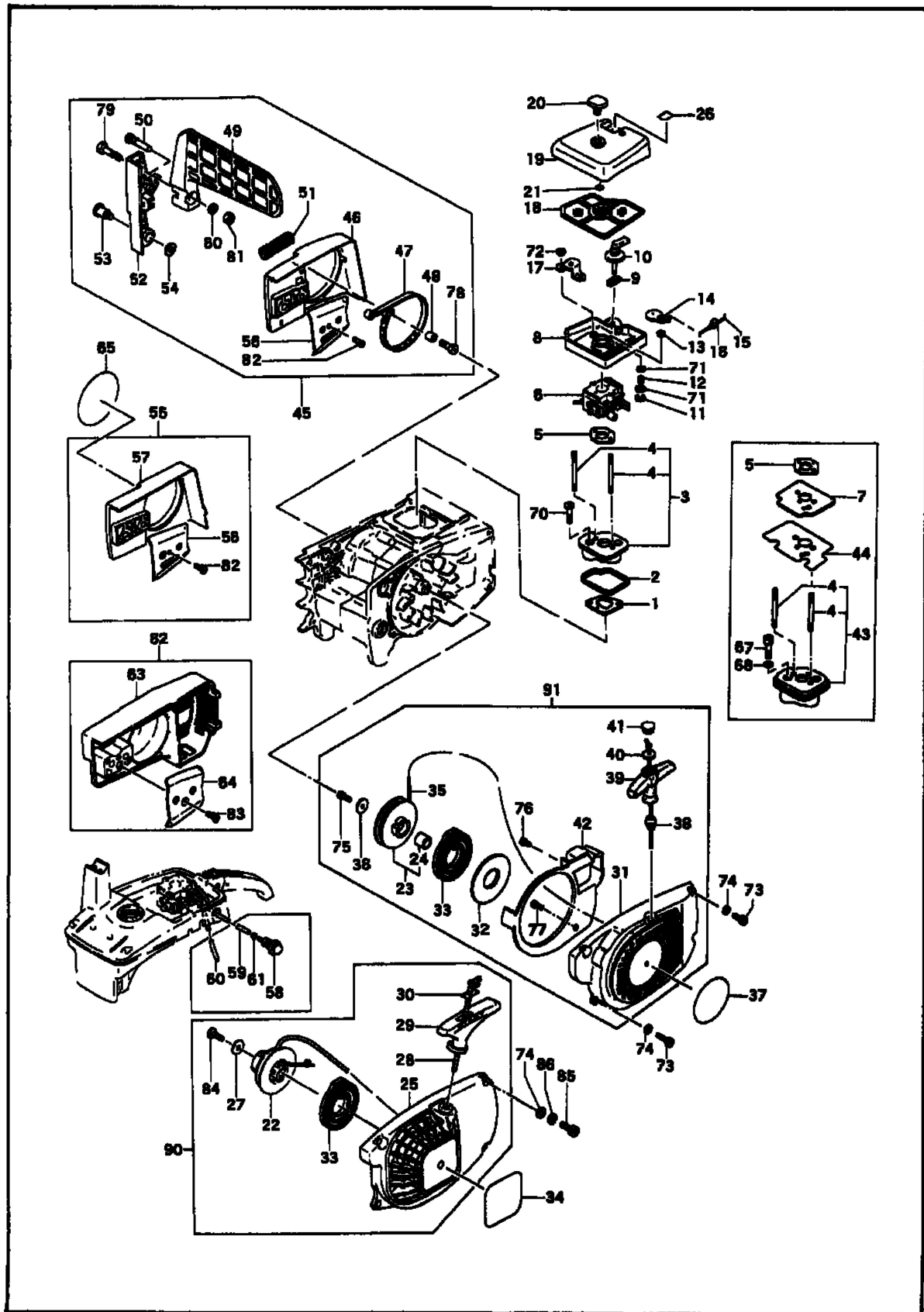
第1図 エンジン外装部 I
