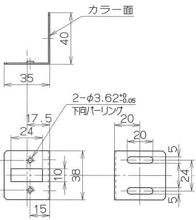
取付ベース
