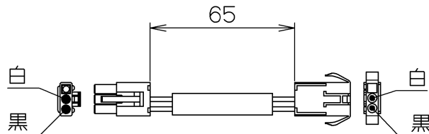
信号線（右側排気変更時に使用）
