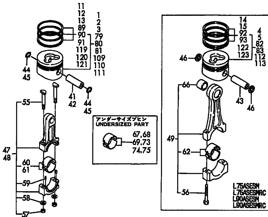
Fig. 6 ピストン&コネクティングロッド PISTON & CONNECTING ROD
